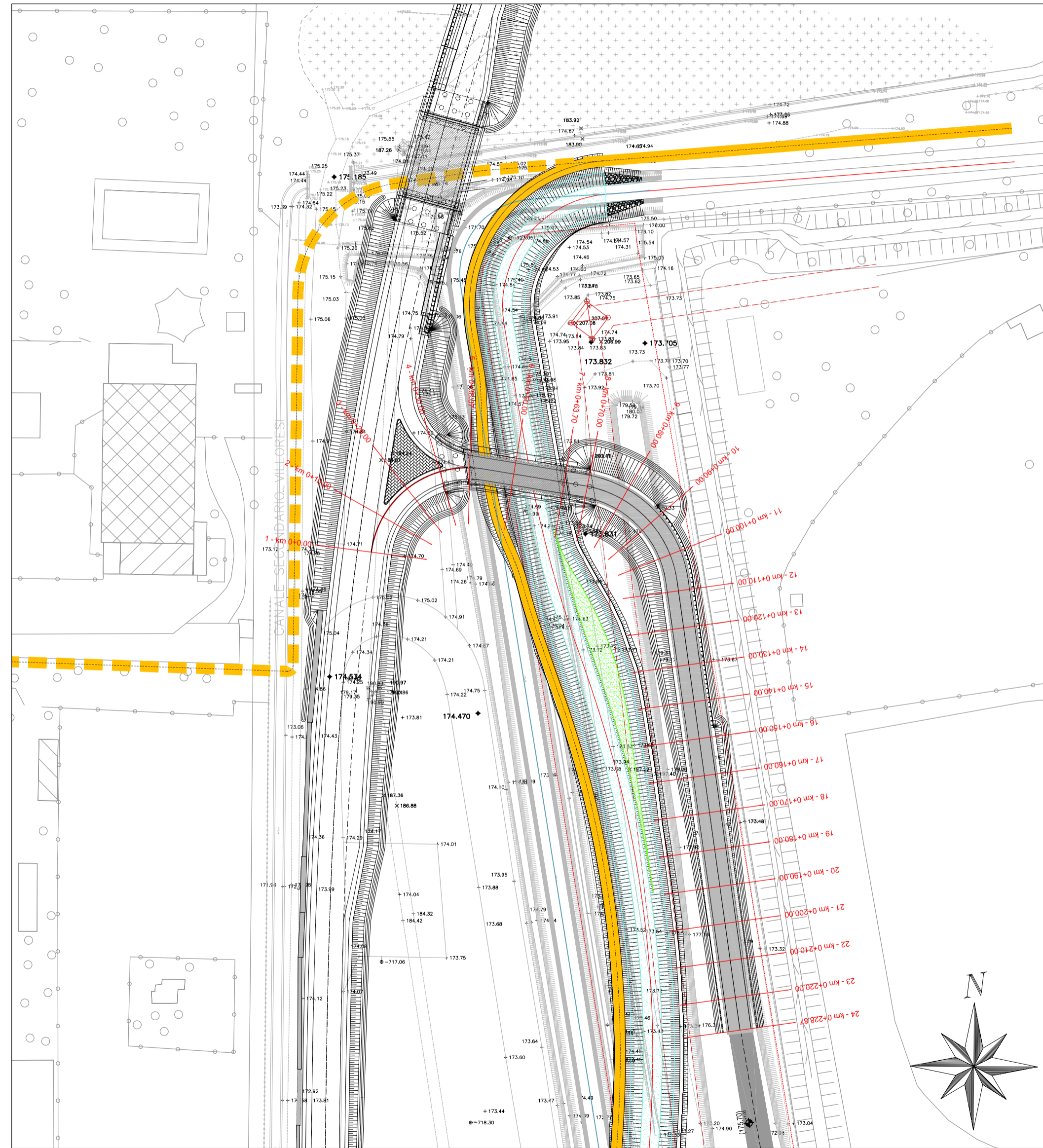
Stralcio planimetrico - Scala 1:1000 -
