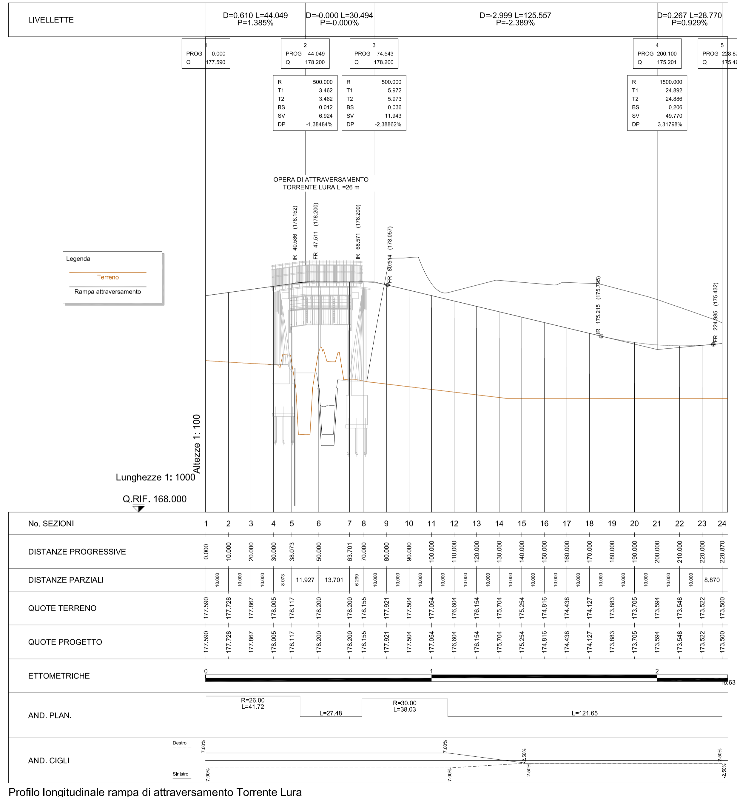
Profilo longitudinale rampa di attraversamento Torrente Lura
