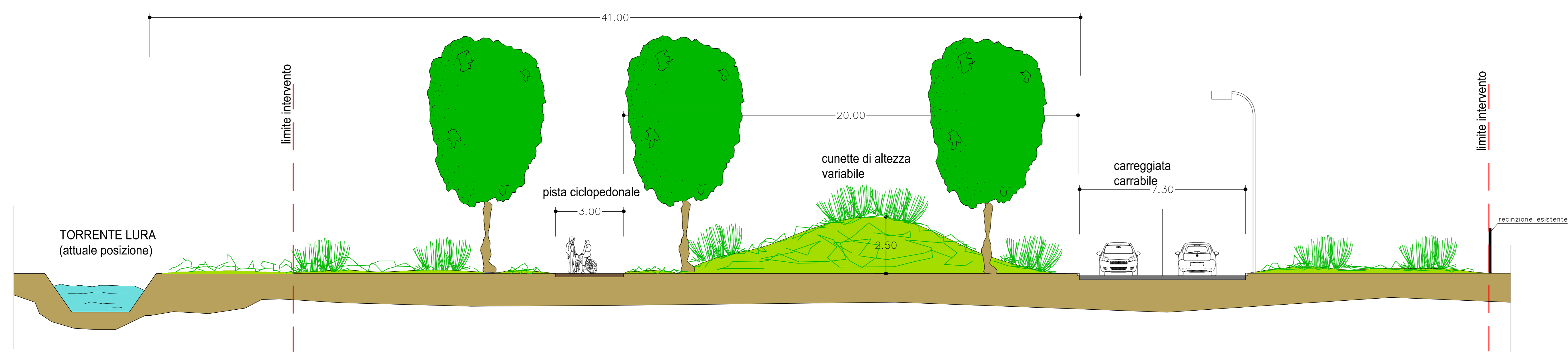
SEZIONE TIPO Viabilità accesso da Nord
