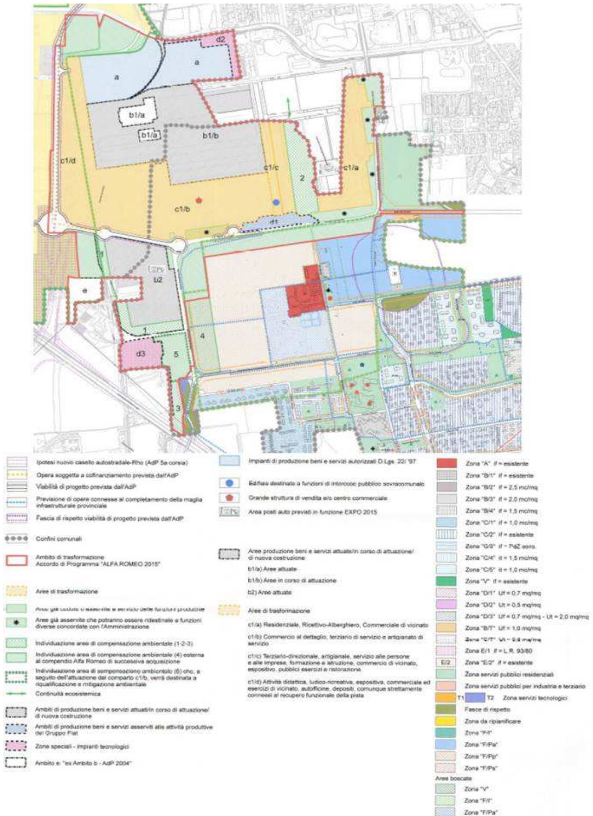
Fig. 39 – Azzonamento dell'AdP per la ripermimetrazione, riqualificazione e reindustrializzazione delle aree ex Fiat - Alfa Romeo nei Comuni di Arese e Lainate
