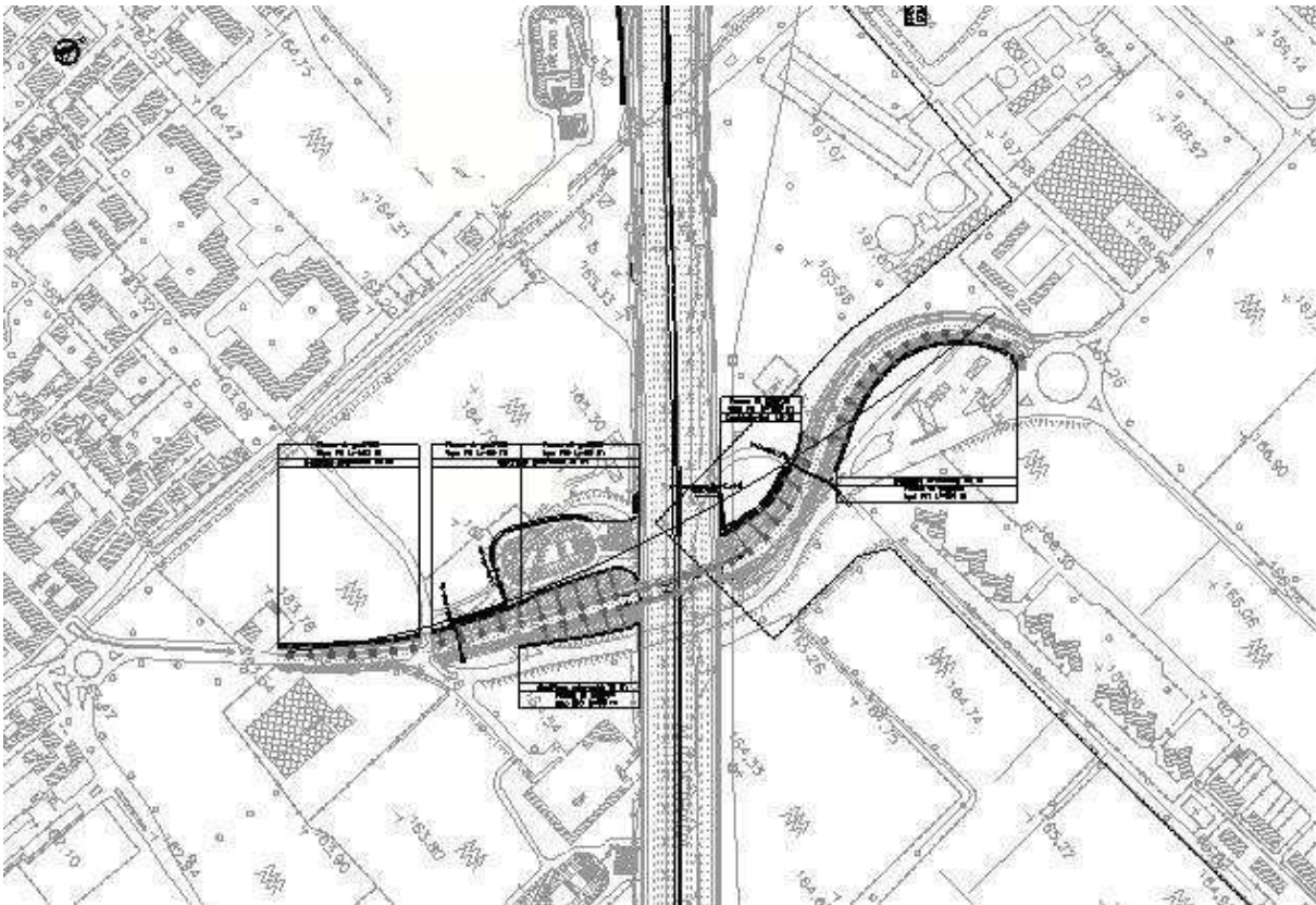
Fig. 33 – Ampliamento quinta corsia dell'Autostrada A8 nel tratto tra la barriera di Milano Nord e il futuro casello di Lainate
